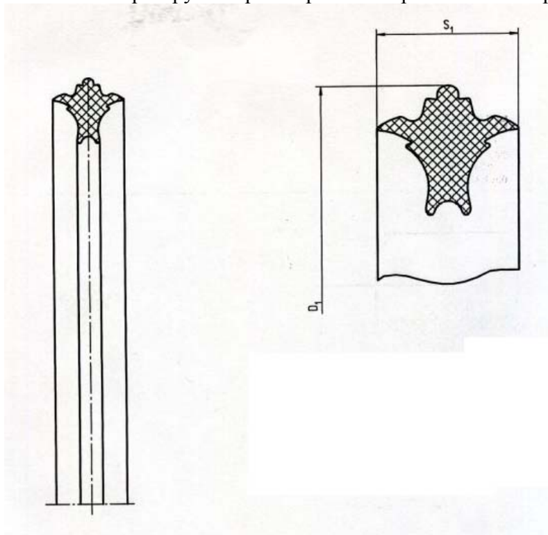
Рисунок В 1. Резиновое кольцо для уплотнения труб.
