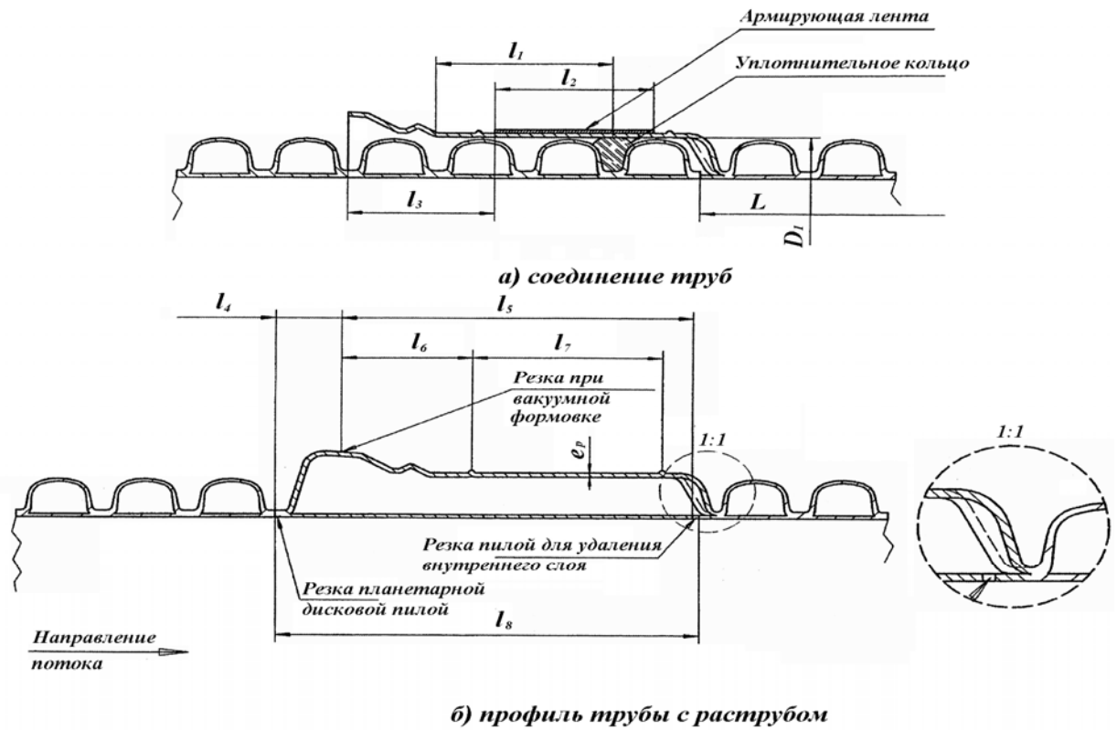
Рисунок 4. Схемы профилей труб номинальным диаметром 300 мм и их соединений.
