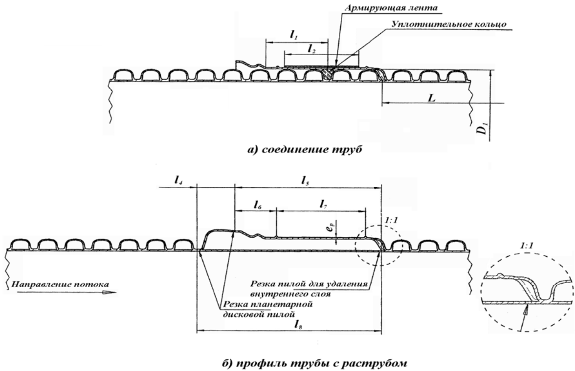
Рисунок 2. Схемы профилей труб номинальным диаметром 200 мм и их соединений
