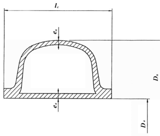
Рисунок 1 Схема полипропиленовой трубы с двухслойной стенкой а) общий вид, б) секция трубного профиля
