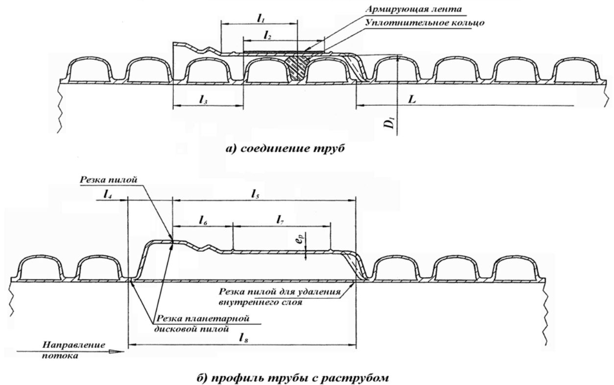
Рисунок 4. Схемы профилей труб номинальным диаметром 300 мм и их соединений.
