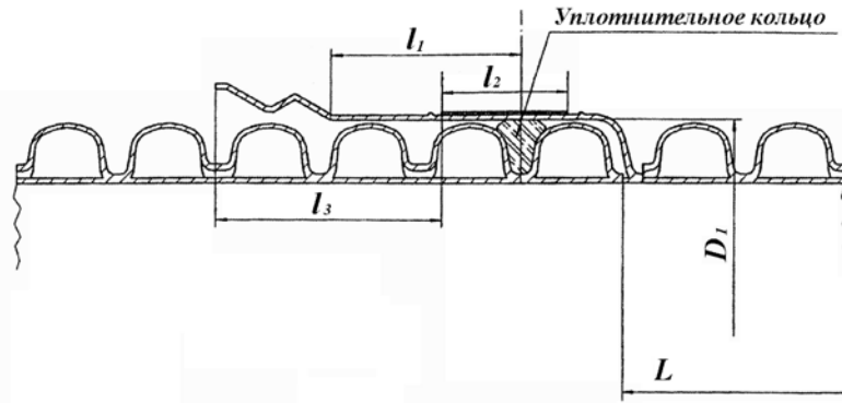
а) соединение труб
