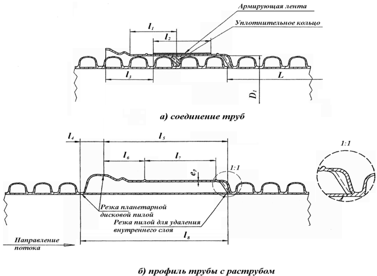
Рисунок 3. Схемы профилей труб номинальным диаметром 250 мм и их соединений.
